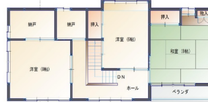
2階平面図
